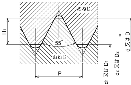
薄鋼電線管ねじ JIS C 8305 : 2019 附属書
