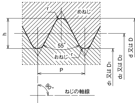
厚鋼電線管ねじ JIS C 8305 : 2019 附属書
