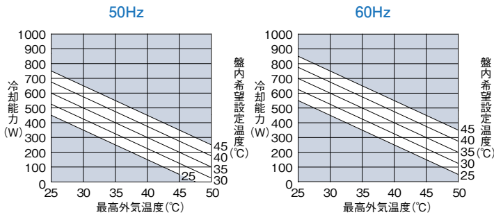
OCA-500BE-100V
