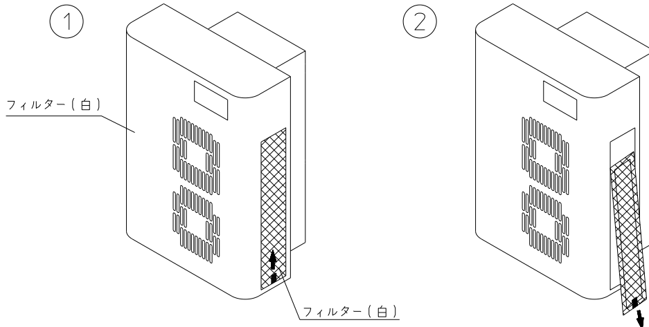
図7-1. フィルタ脱着方法
