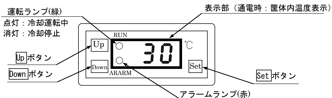
図4-1. 操作パネル各部名称
