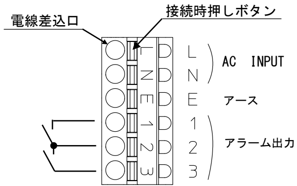
図3-1. 端子台詳細図
