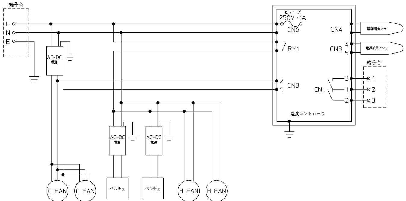
◎00E-200FSC-A1 回路図（例）
