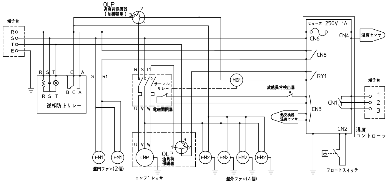
◎ OCA-S2300AC-A200 電気回路図
