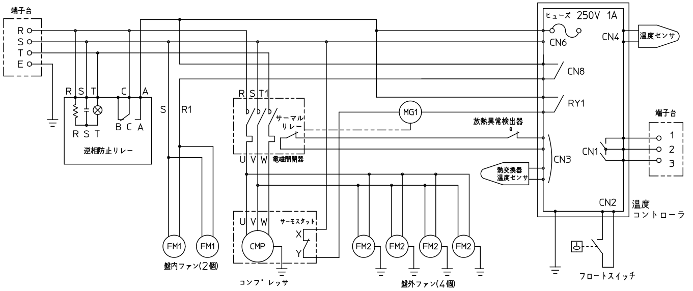
◎ OCA-S3000AC-A200 電気回路図
