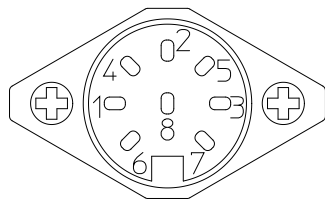
コネクタピン位置 本体コネクタ結合面視 Connector pin arrangement on Main body side view
