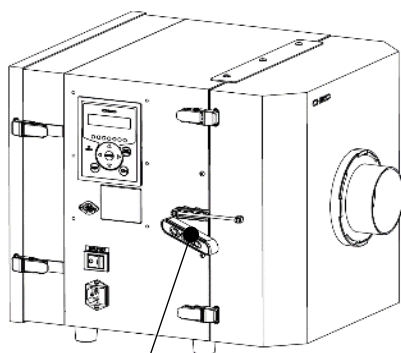
外部圧カバー External pressure cover
