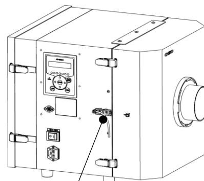
外部圧検出用チューブ External pressure detection tube
